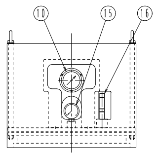
A-A矢視
