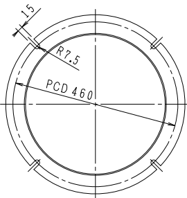
アンカーボルト取付詳細図
